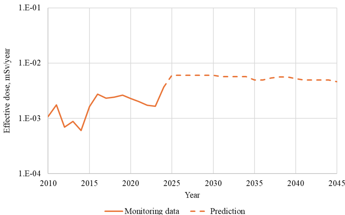
Рисунок 4-3. Годовая эффективная доза облучения населения в результате вывода из эксплуатации ИАЭС; — данные мониторинга; - - прогноз
